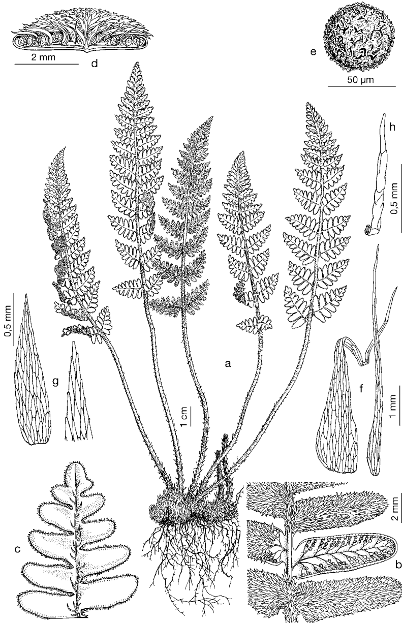
Lám. 17.— Notholaena marantae subsp. marantae , Anoia, Barcelona (BC 149207): a) hábito; b) detalle del envés de una pinna, a una de las pínulas se han retirado las páleas y muestra los esporangios; c) detalle del haz de una pinna; d) corte transversal de una pínula; e) espora en vista distal; f) páleas del rizoma; g) páleas del envés de las pínulas; h) pelo del envés de las pínulas.
